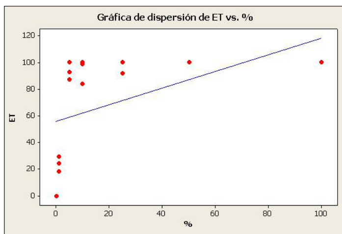
Gráfico 2. Análise de regressão linear com os parâmetros de eficiência do tratamento (ET) (x) e concentração da tintura de Cymbopogon nardus (%) (y) em teleóginas de Rhipicephalus (Boophilus) microplus , Santa Maria, RS.
