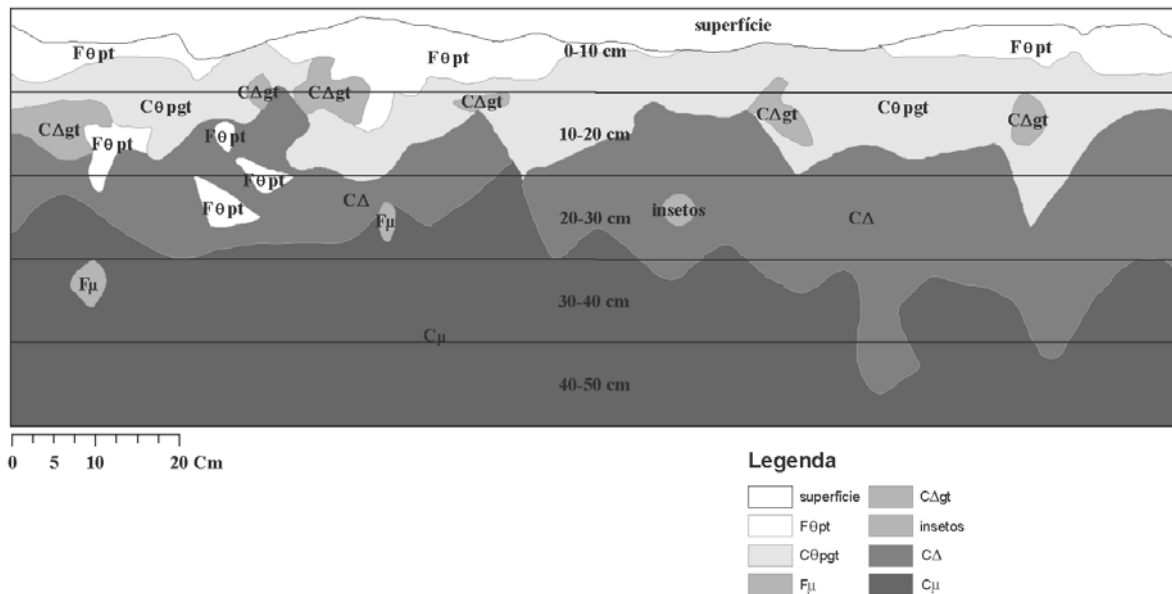
Figura 1. Esquema demonstrativo dos planos de informação “perfil” e “profundidade”, sobrepostos. (F = volume de solo fissurado; C = volume de solo contínuo; Δ = torrões compactados; μ = torrões porosos; Ø = intermediário entre Δ e μ; pt = pequenos torrões; gt = grandes torrões; pgt = presença de pt e gt).
